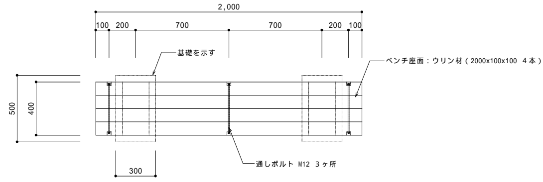
《 平面図 S=1/20 》
