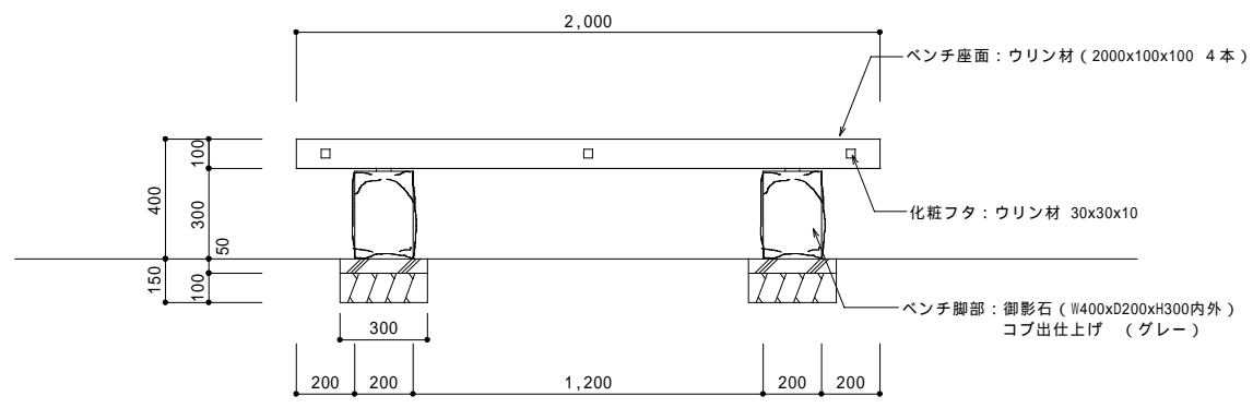
《 正面図 S=1/20 》
