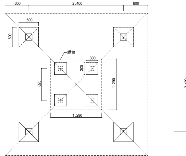
《 平面・基礎 伏せ図 S=1/40 》
