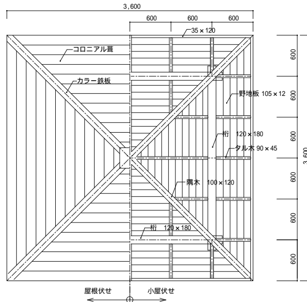
《 屋根・小屋 伏せ図 S=1/40 》
