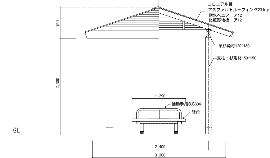
《 正面図 S=1/40 》
