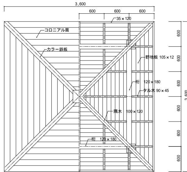
《 屋根・小屋 伏せ図 S=1/40 》
