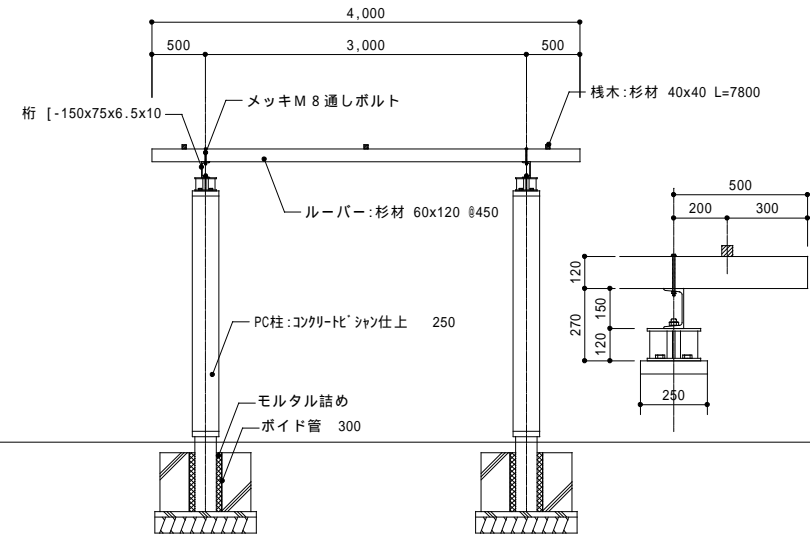
《 断面図 S=1/50 》
