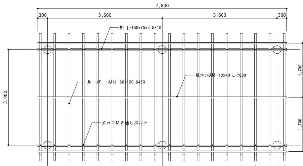
《 平面図 S=1/50 》
