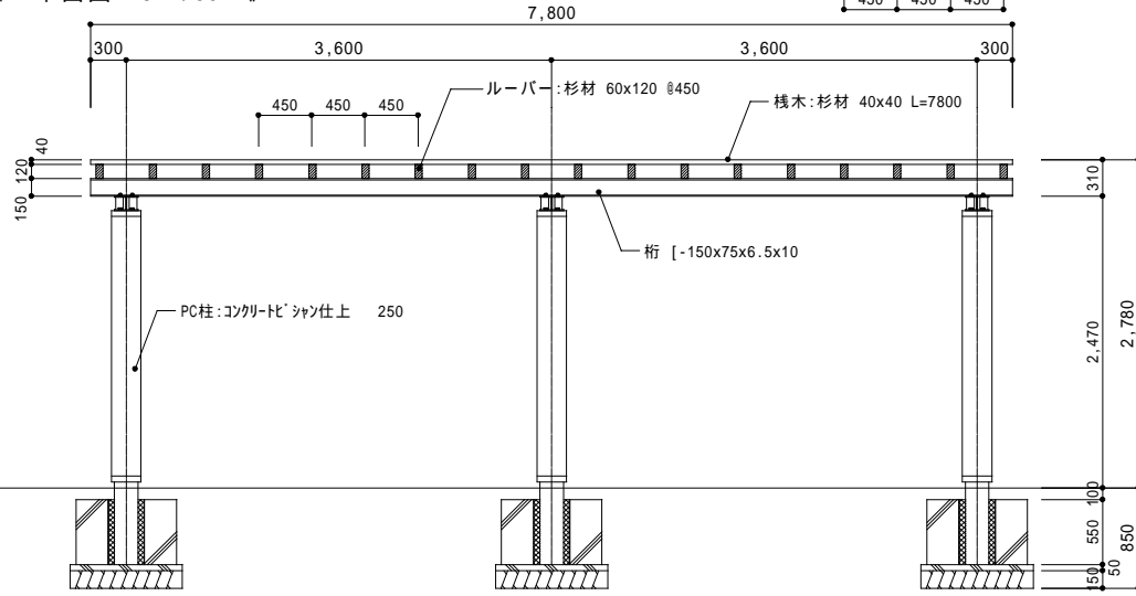
《 立面図 S=1/50 》
