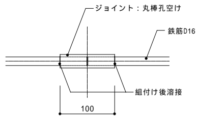
《 ジョイント部詳細図 S=1/5 》
