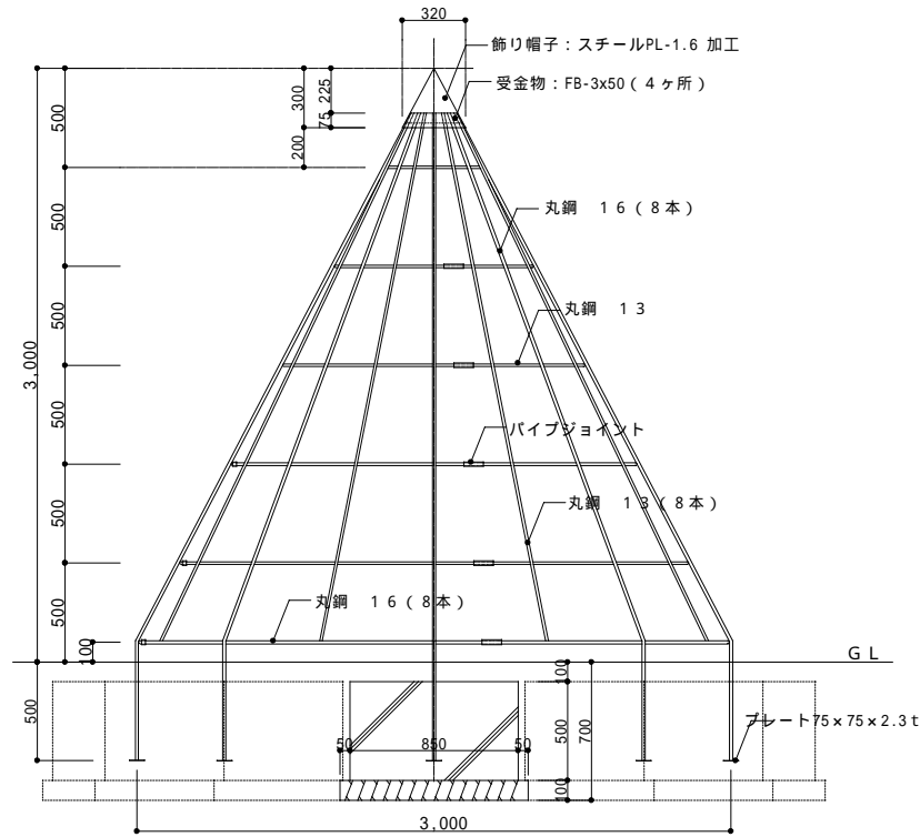
《 断面図 S=1/30 》
