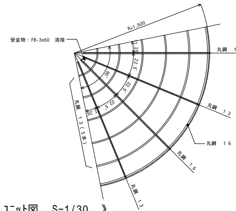
《 ユニット図 S=1/30 》
