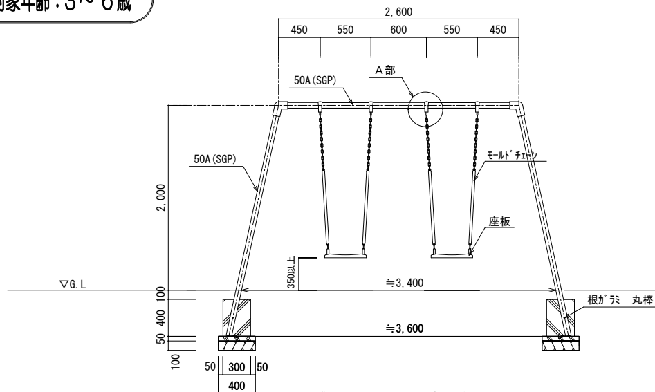
《 正面図 S=1/40 》
