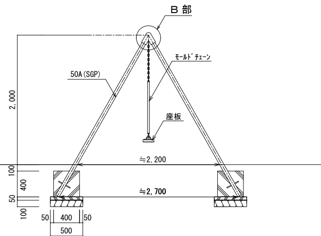
《 側面図 S=1/40 》
