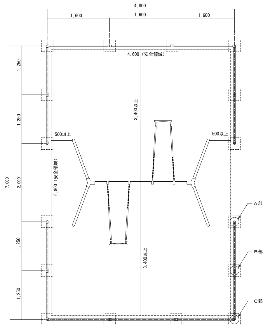
《 平面図 S=1/40 》
