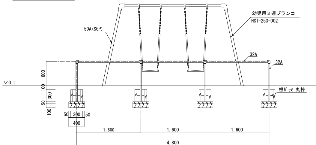
《 正面図 S=1/40 》
