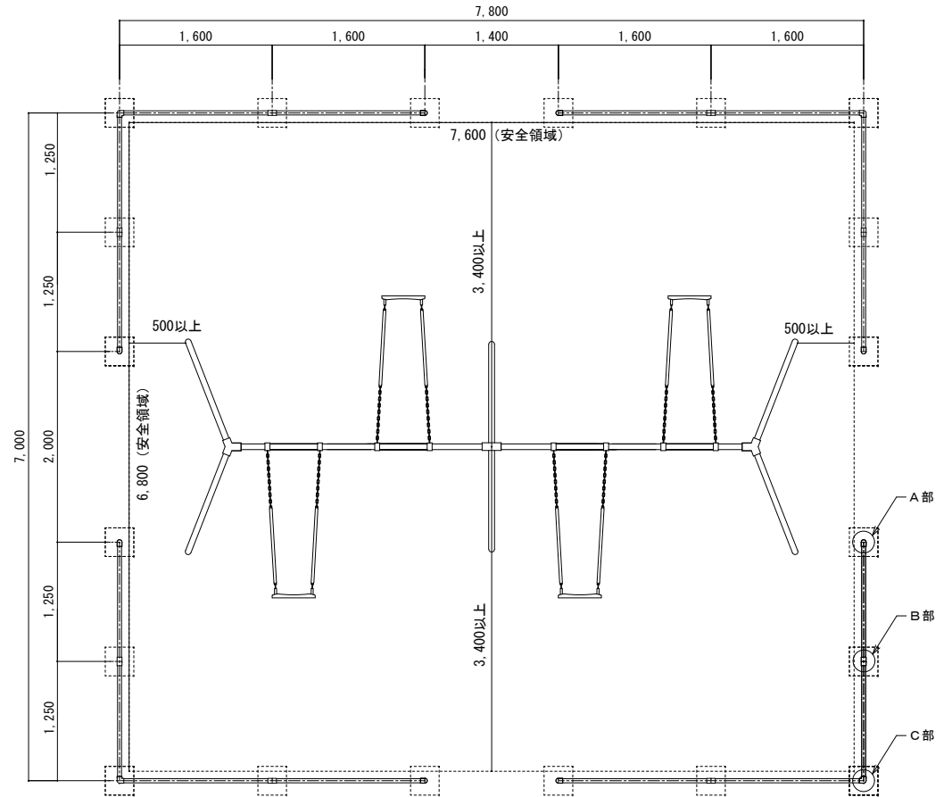
《 平面図 S=1/50 》
