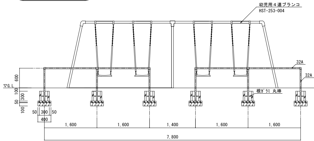
《 正面図 S=1/50 》
