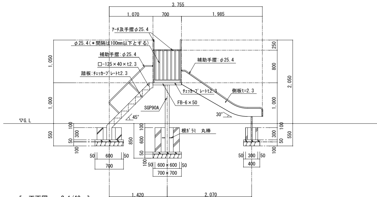
《 正面図 S=1/40 》
