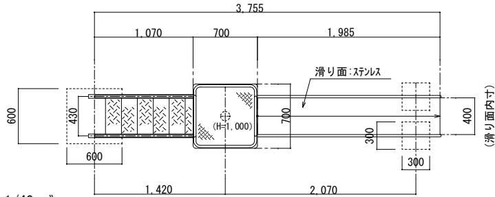
《 平面図 S=1/40 》
