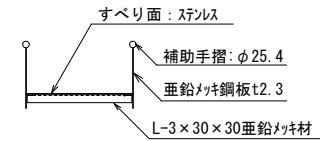
《 すべり面詳細図 S=1/20 》
