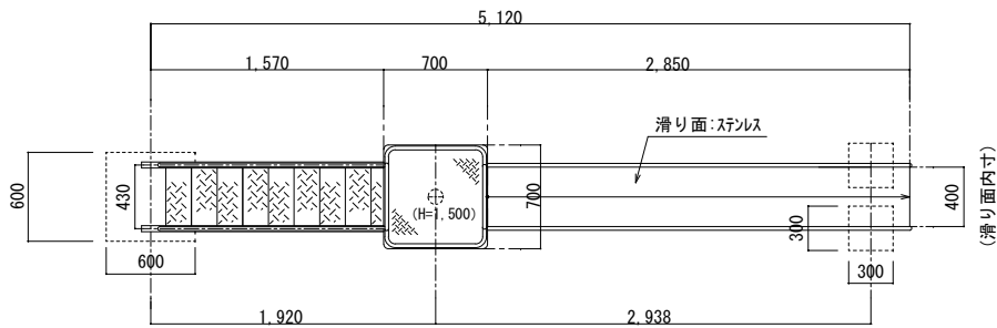
《 平面図 S=1/40 》
