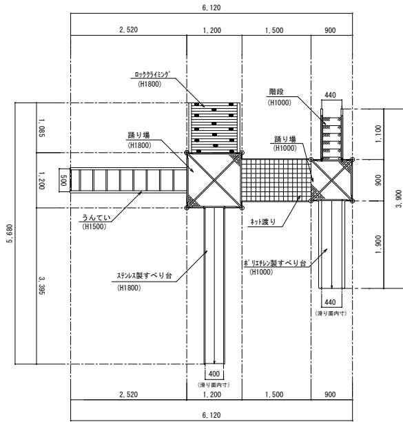
《 平面図 S=1/80 》
