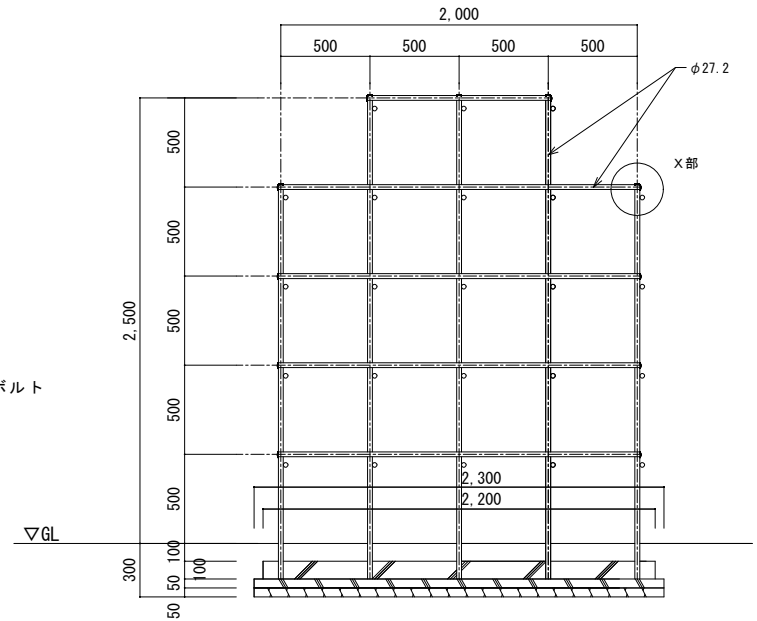
《 断面図 S=1/30 》
