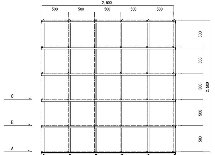
《 平面図 S=1/30 》
