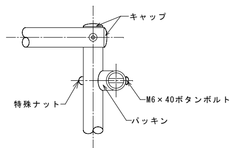
《 X部詳細図 》
