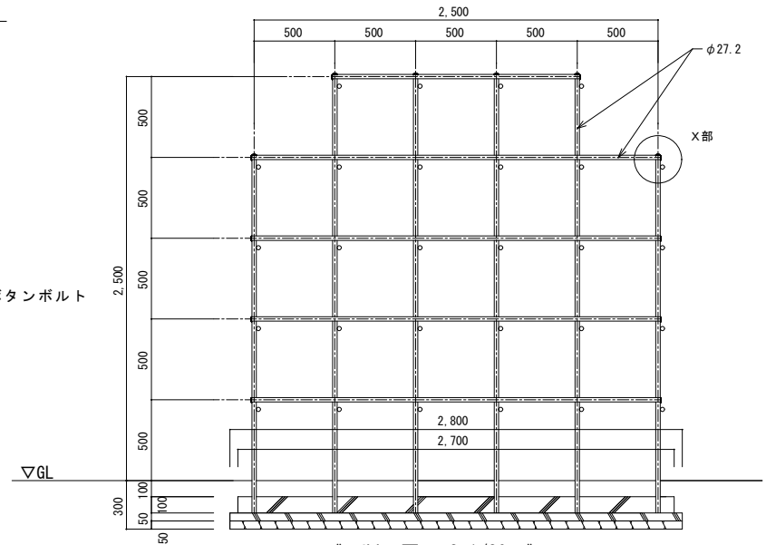
《 断面図 S=1/30 》
