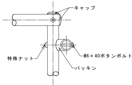
《 X部詳細図 》
