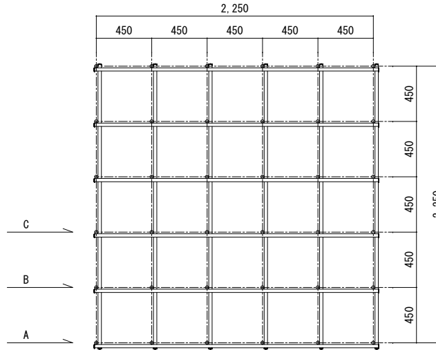
《 平面図 S=1/30 》
