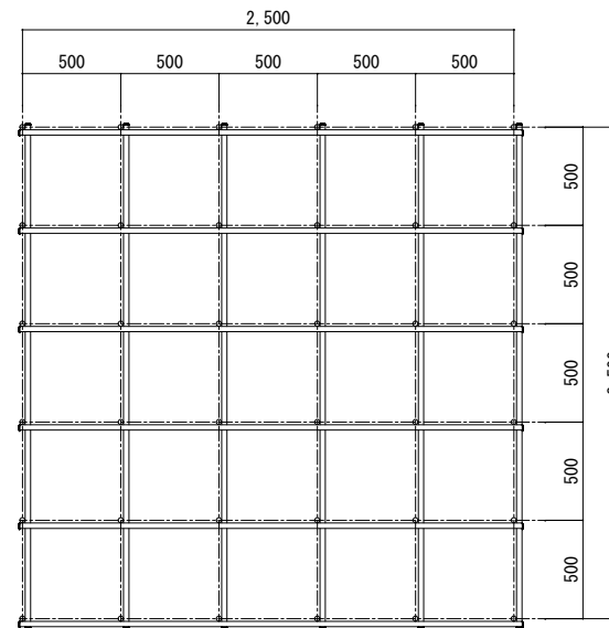
《 平面図 S=1/30 》
