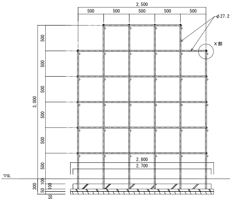
《 断面図 S=1/30 》
