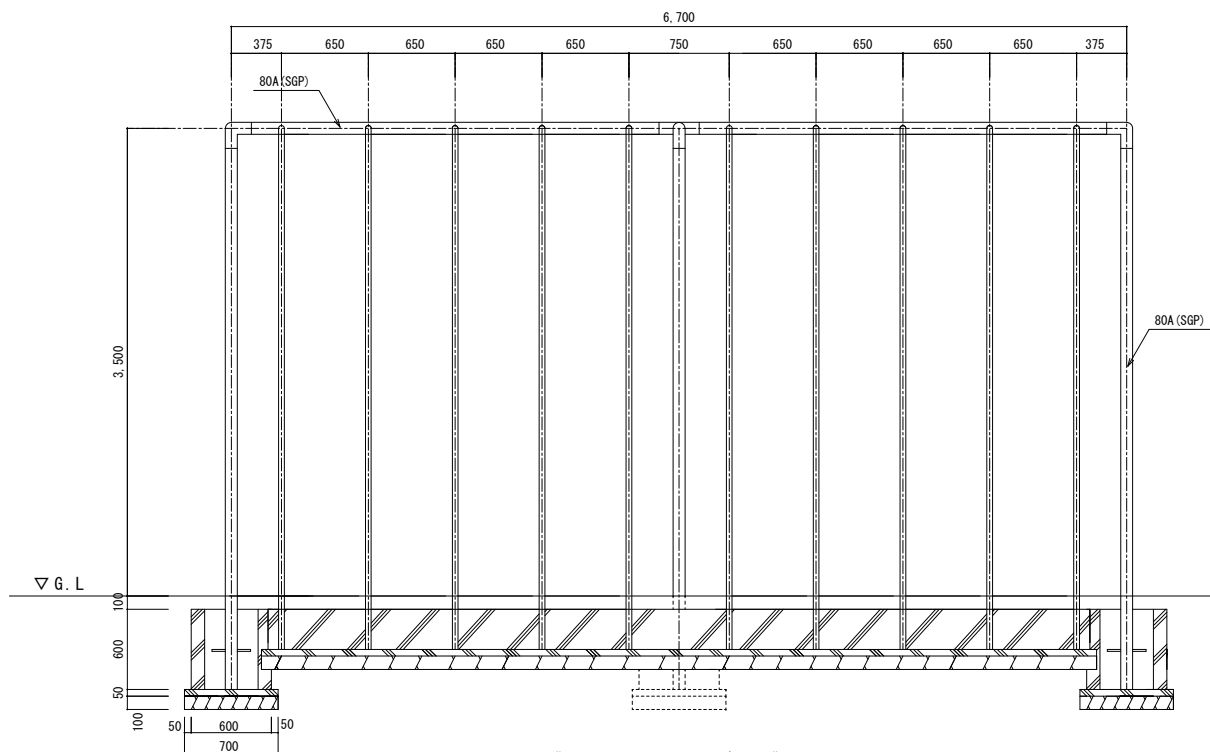
《 正面図 S=1/40 》
