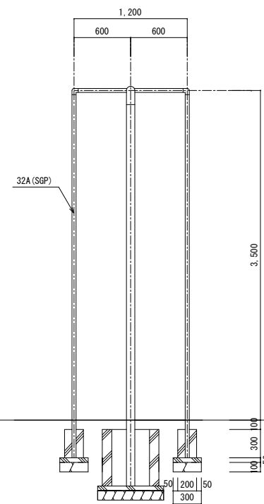
《 側面図 S=1/40 》
