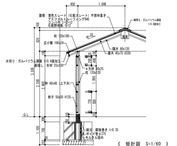
《 矩計図 S=1/60 》
