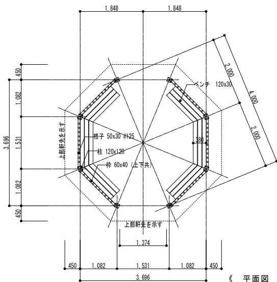
《 平面図 S=1/80 》
