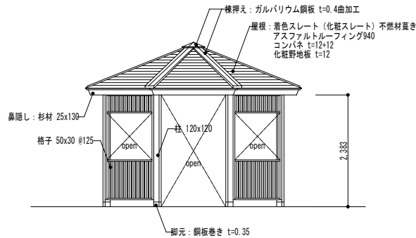
《 立面図 S=1/80 》
