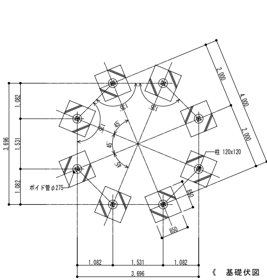
《 基礎伏図 S=1/80 》
