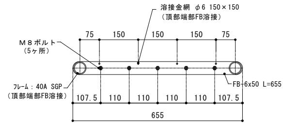
《 接続部詳細図 S=1/10 》
