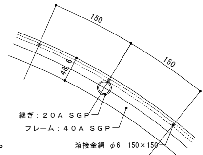
《 詳細図 S=1/5 》
